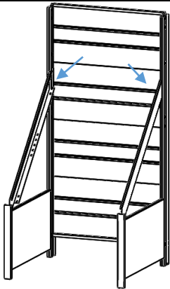
Encastre de las vigas laterales.
